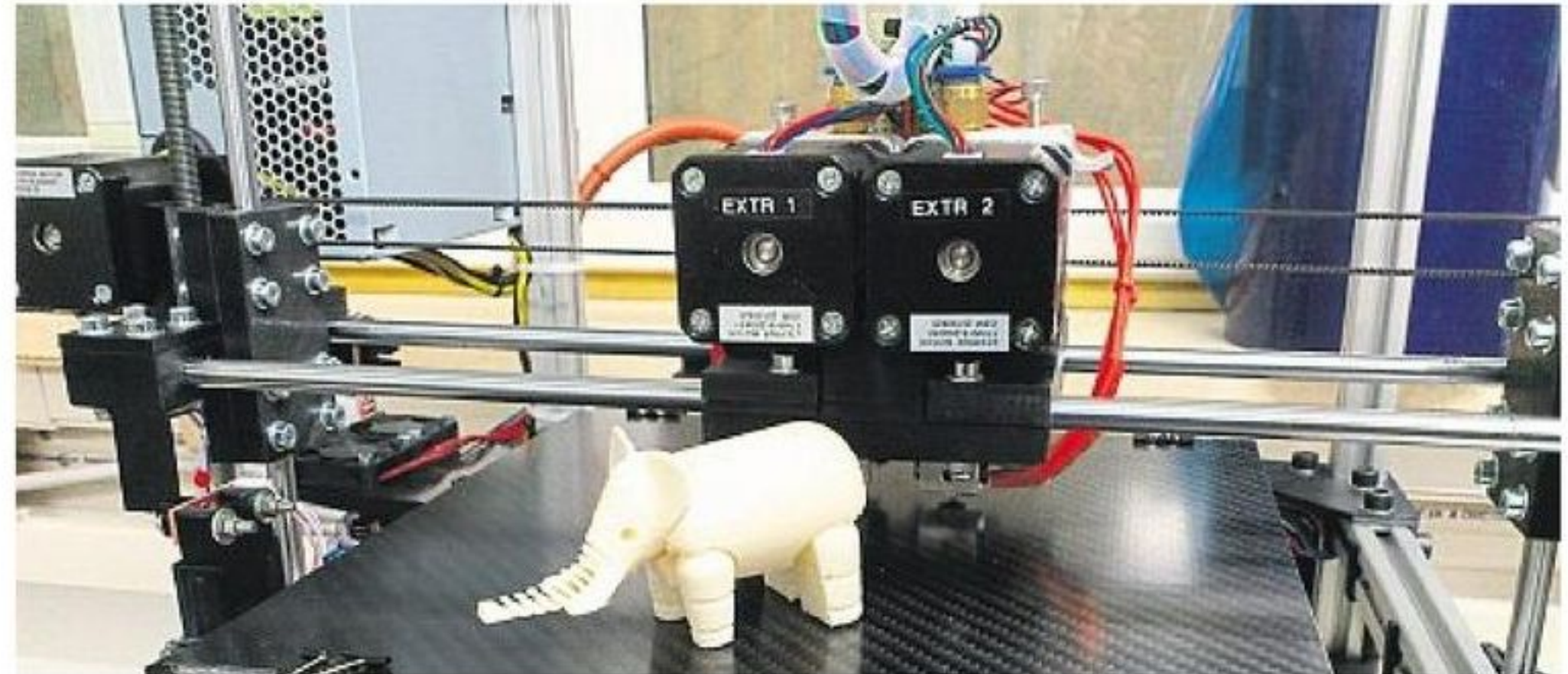
Der MCSM Modellbau-Club hat in Eigenregie einen 3D Drucker entwickelt und gebaut. Foto: oh
